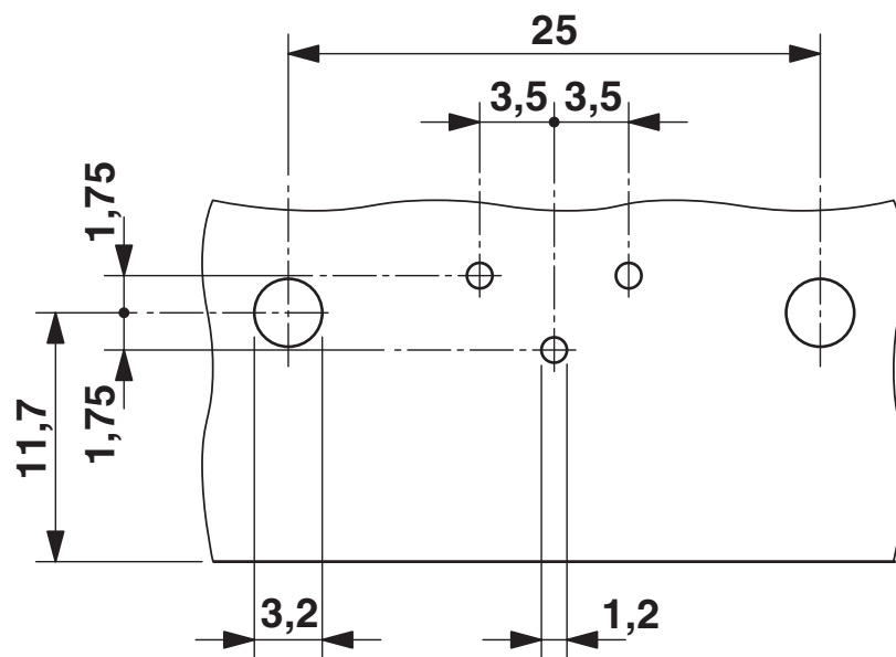
Bohrplan/Lötpadgeometrie
