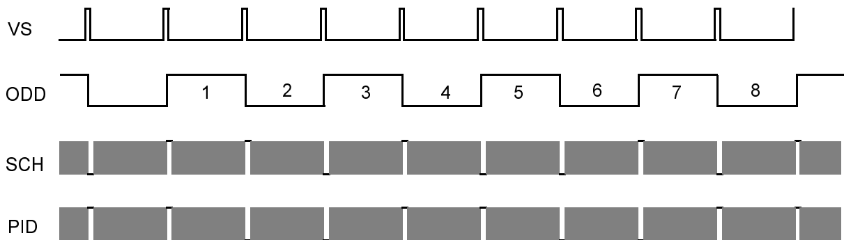
Truth Table
