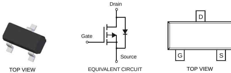
SOT-23
