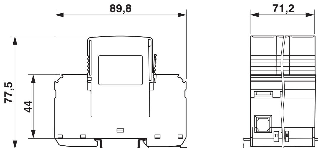
尺寸图
