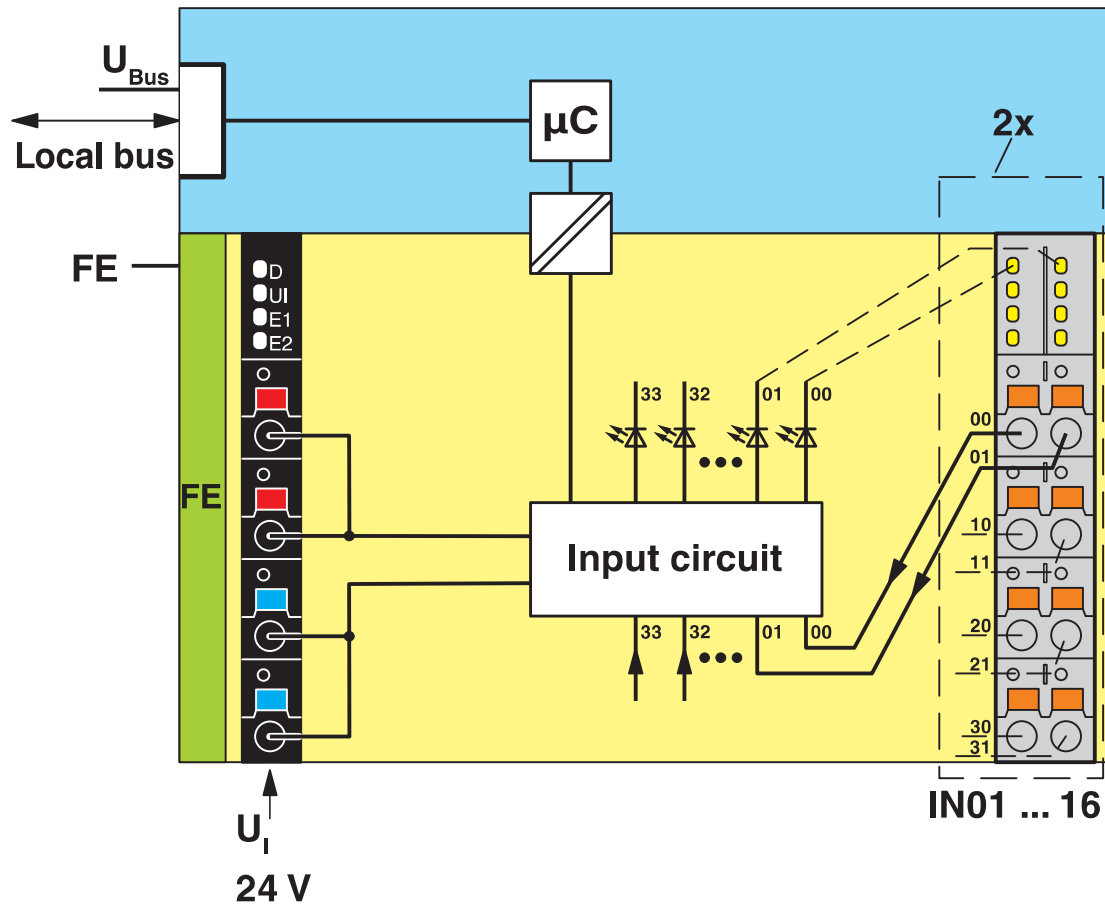
结构框图
