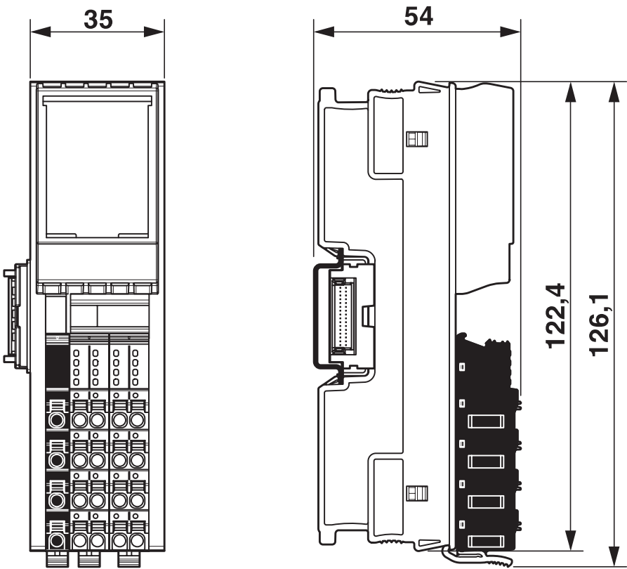
尺寸图
