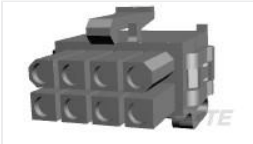
TE Part #794245-1 08P MINI UMN2 PLUG HSG UL94V2
