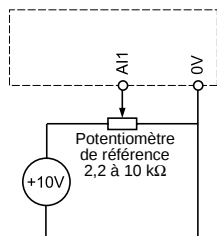
Entrée analogique Utilisation 10 V externe
