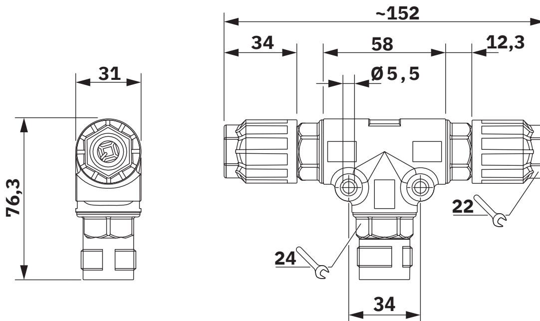
Maßzeichnung
