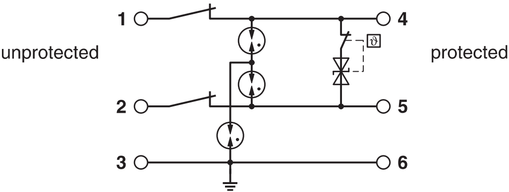
电路图
