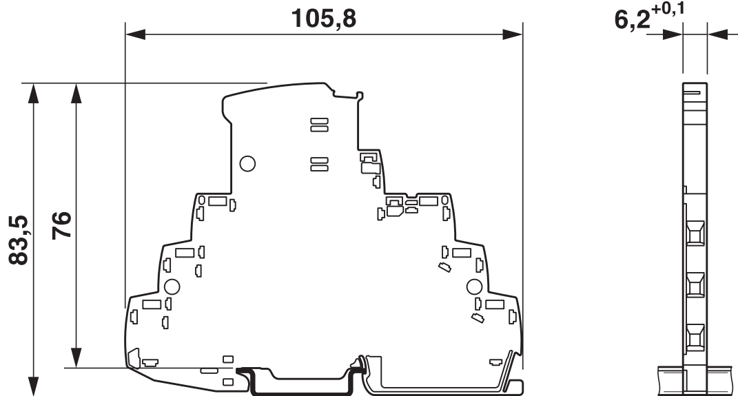
尺寸图
