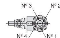
Disposition des broches du connecteur mâle
