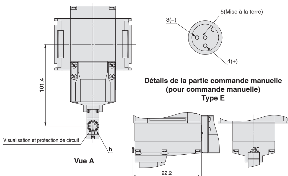
Figure détaillée de la section b du connecteur M12
