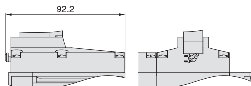
Détails de la partie commande manuelle (pour commande manuelle) Type E
