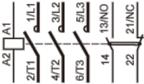
1NO+1NC(LANN11)
