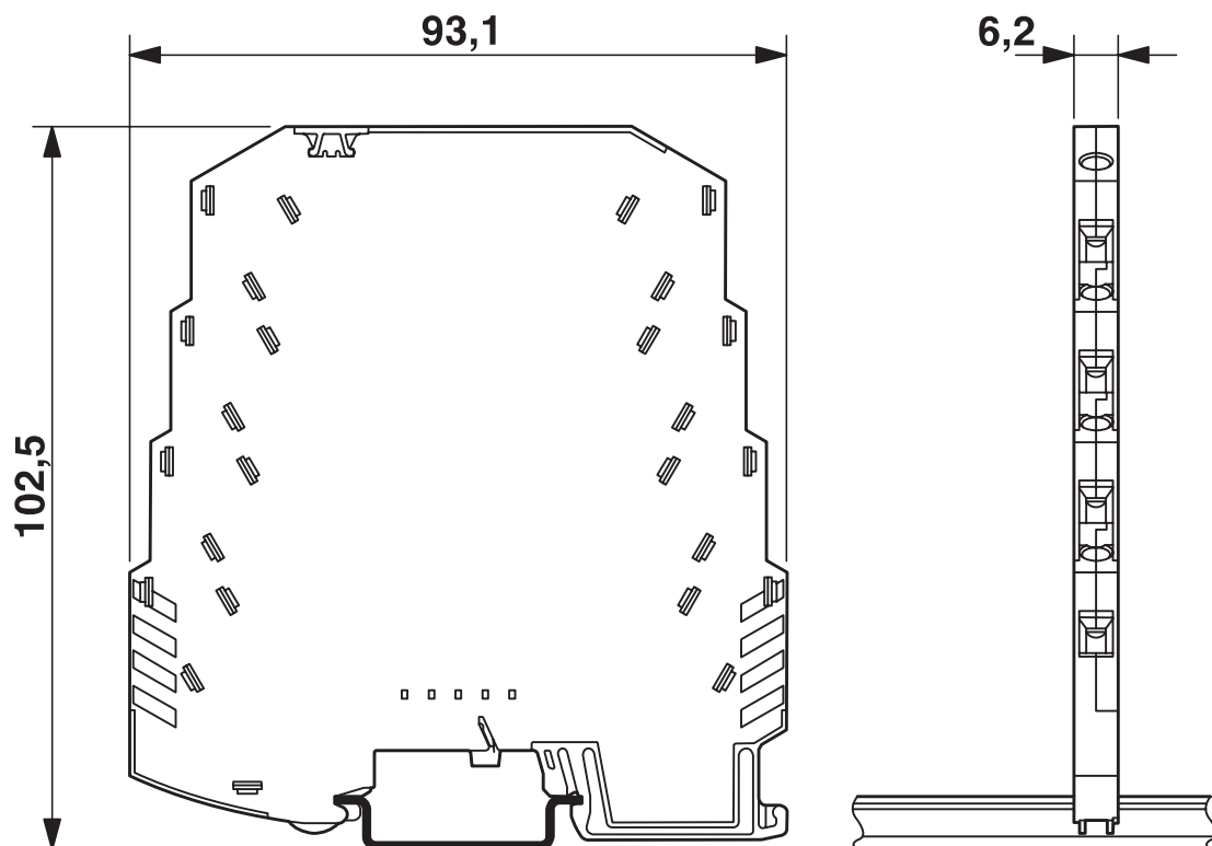
尺寸图
