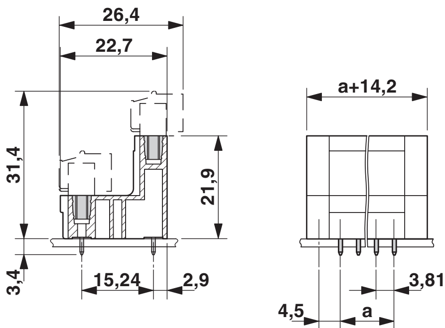
尺寸图
