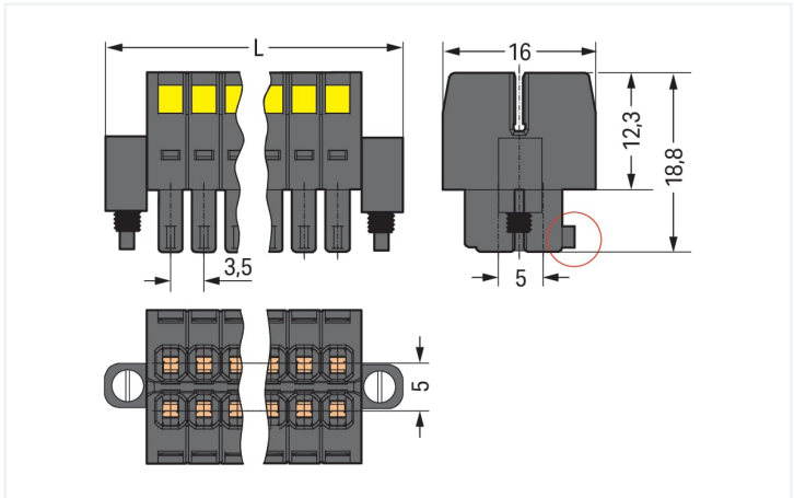
Dimensions en mm L = [( \text{nombre de pôles} / 2 ) - 1] \times \text{pas} + 13,6 \text{ mm} (cercle rouge) tige de codage
