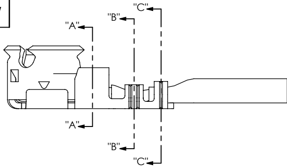
MH081-MH1RP
