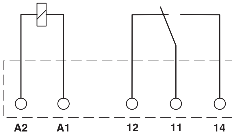
电路图
