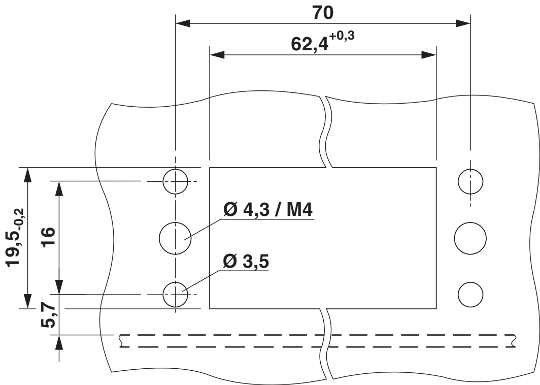
尺寸图
