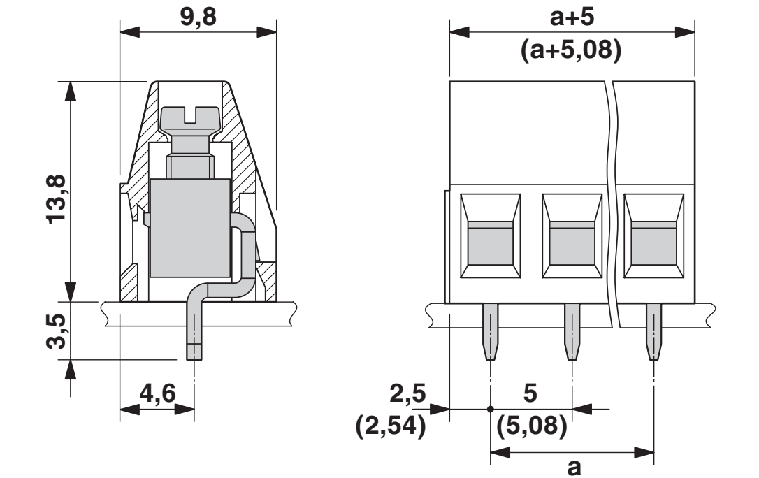
尺寸图
