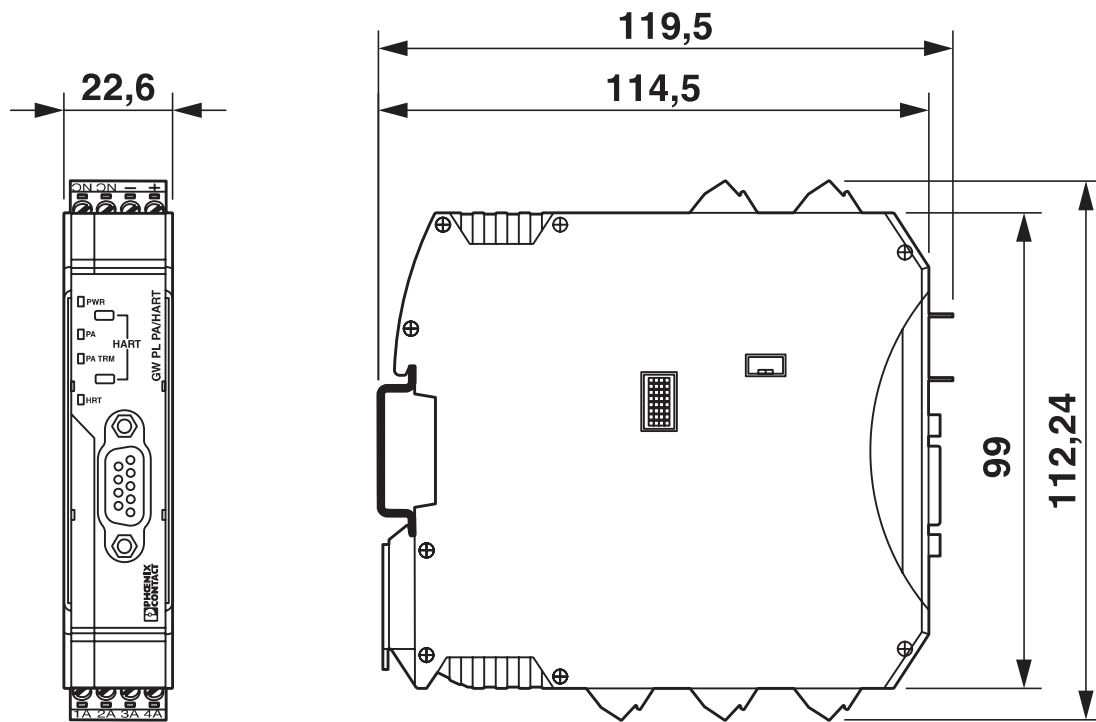
尺寸图
