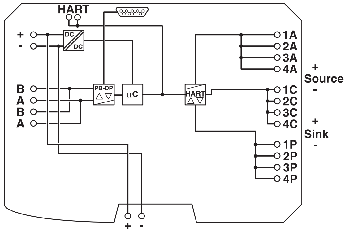
结构框图
