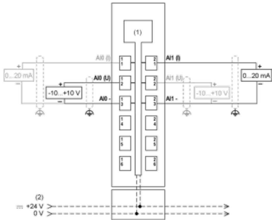
接线图
