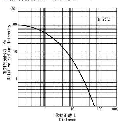
■相対発光出力／距離特性 P_0/L^{\times 1}
