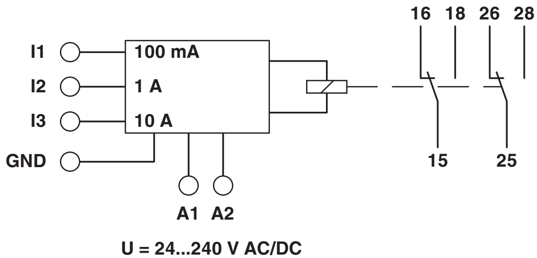
Blockschaltbild
