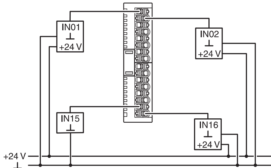
接线图
