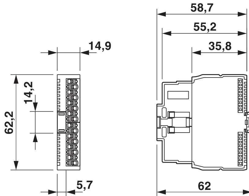
尺寸图
