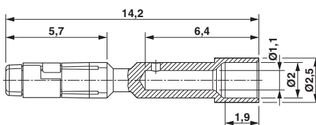
Dessin coté
