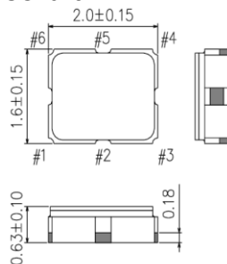
SG2016EHN
