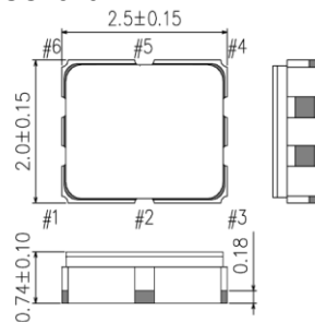
SG2520EHN
