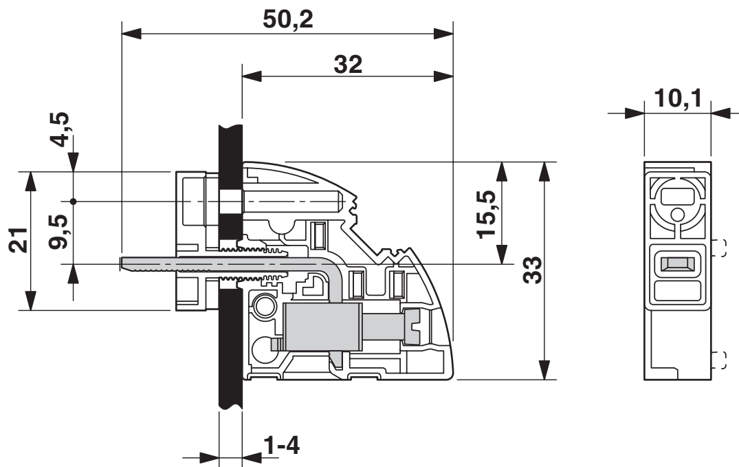
尺寸图
