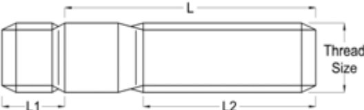
DIN 938
