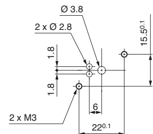
Dimensioni di lavorazione della base
