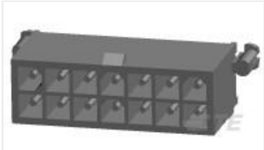
TE Part #1-794074-0 14P MINI UMNL HDR W/O DH SN LF
