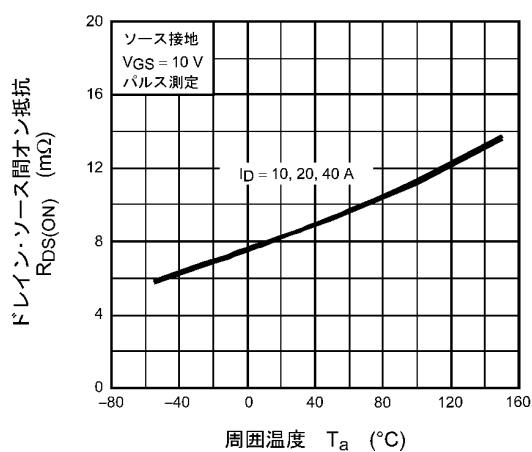
図 8.6 R_{DS(ON)} - T_a
