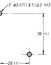
取り付け穴加工寸法
