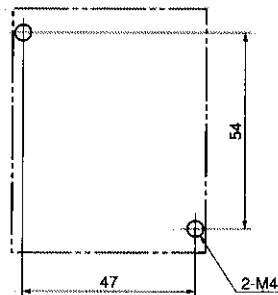
取付穴明寸法
