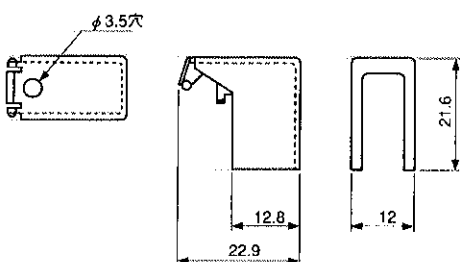
CP-T4主回路用
