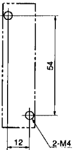
取付穴明寸法
