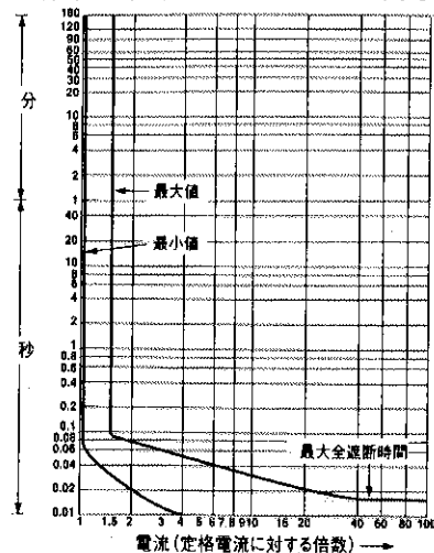
●瞬時形 (I) AC50/60Hz、DC両方
