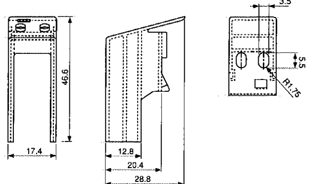
CP-T5主・補助一括用
