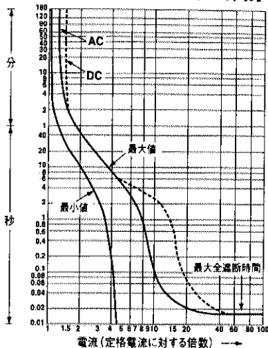
●中速形 (M) AC50/60Hz、DC両方
