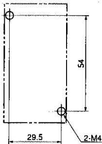
取付穴明寸法
