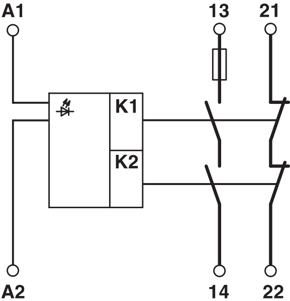
电路图
