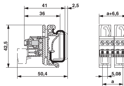
Dessin coté
