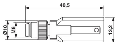
外形寸法
