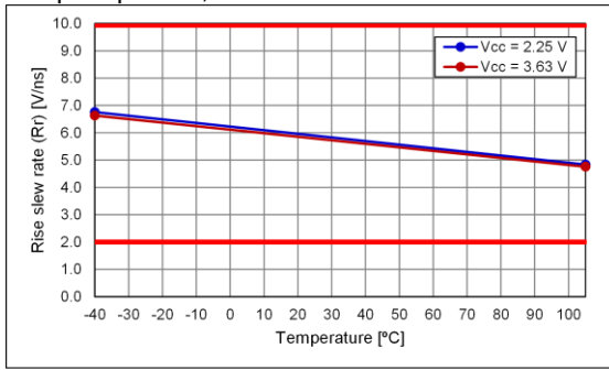
Output option:A, Rise Slew Rate
