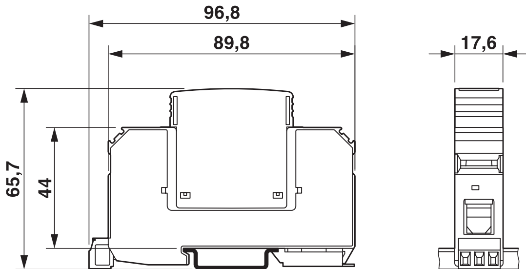
尺寸图
