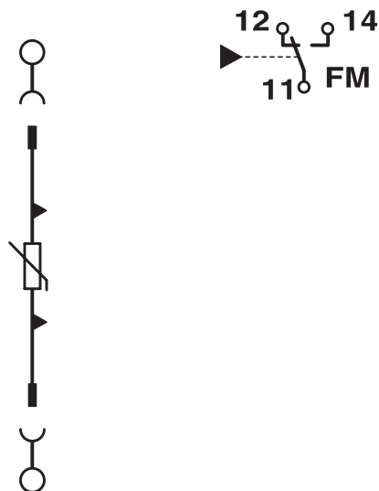
电路图
