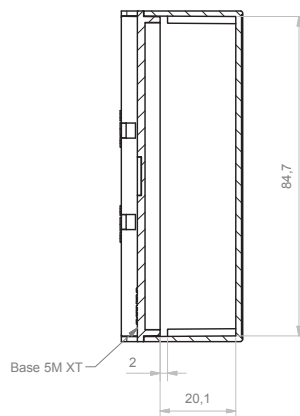
A-A (1 : 1)
