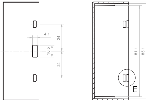
B-B (1 : 1)
