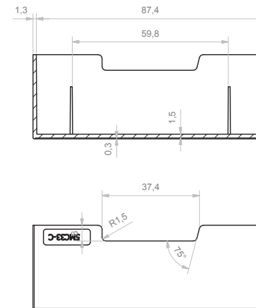
C-C (1 : 1)
