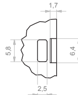
E (2 : 1)
