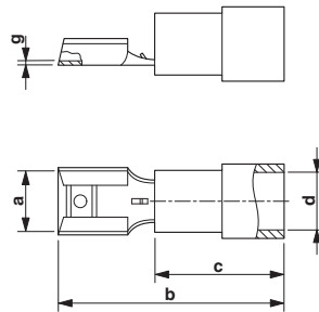
Dessin coté
