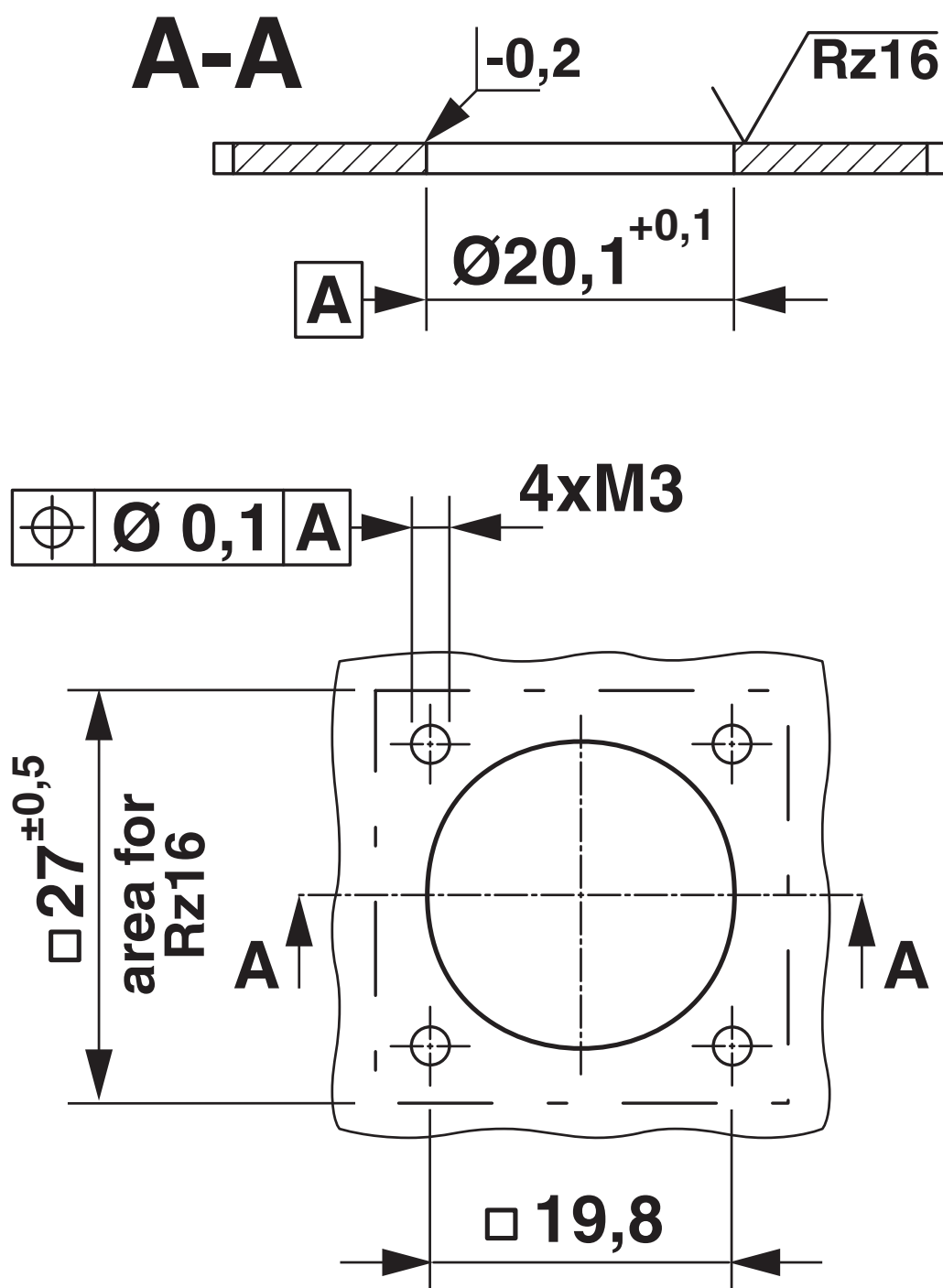
尺寸图
