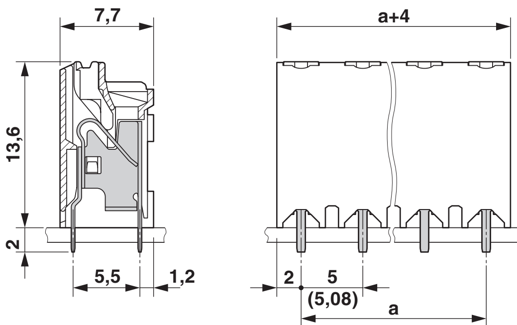
尺寸图
