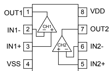
SOP8
