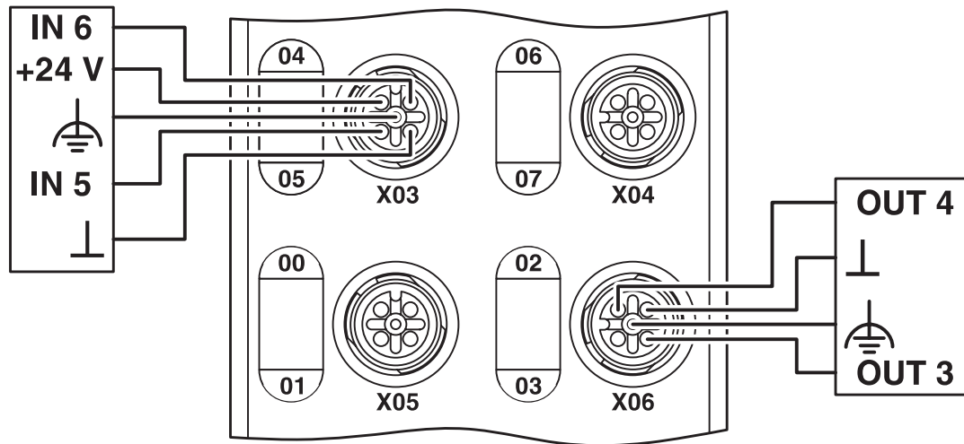
接线图
