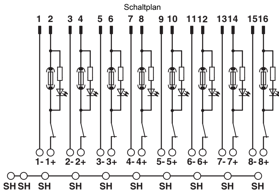
Anschlussbild UM-DELTAV/A/SI/BFI/TP
