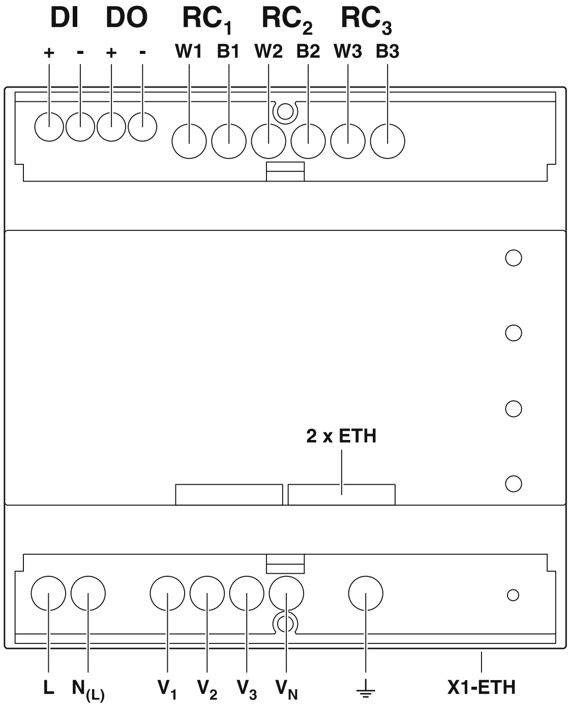
接线图
