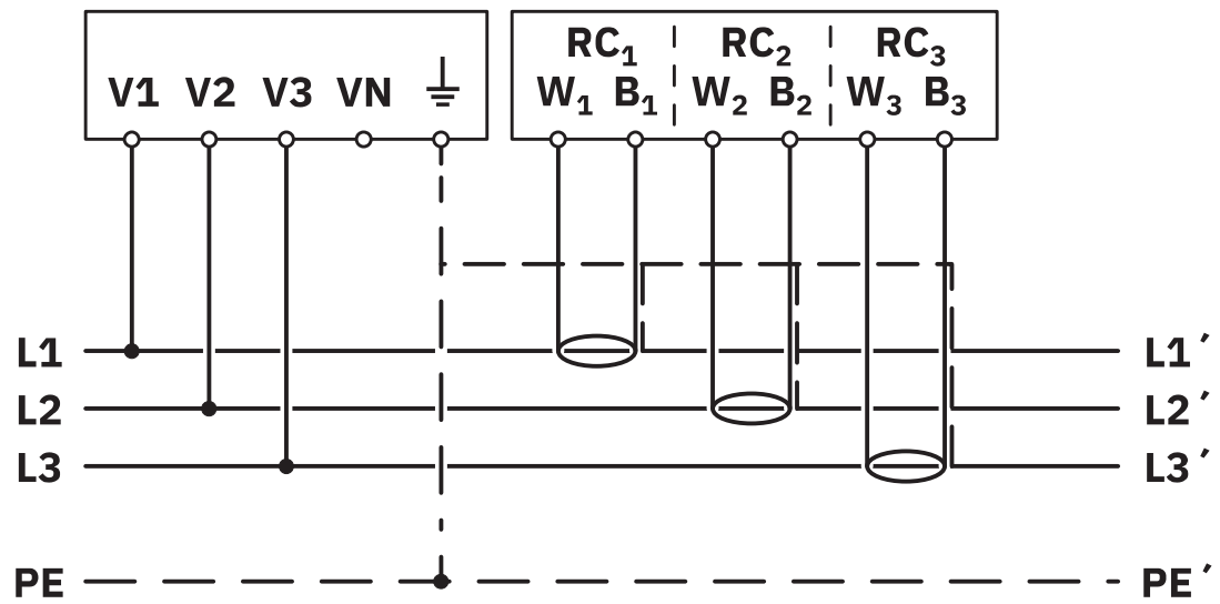
接线图
