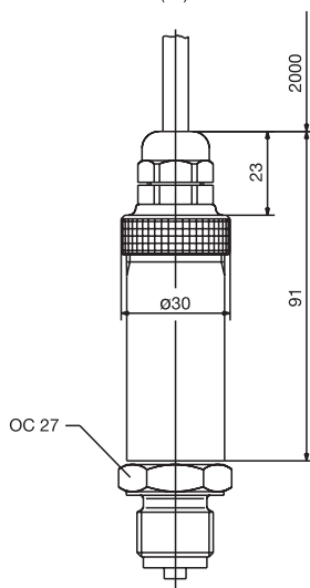
Raccordement électrique avec câble fixe (12)
