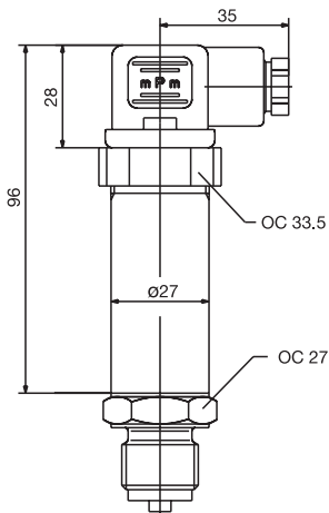
Raccordement électrique avec connecteur (61)
