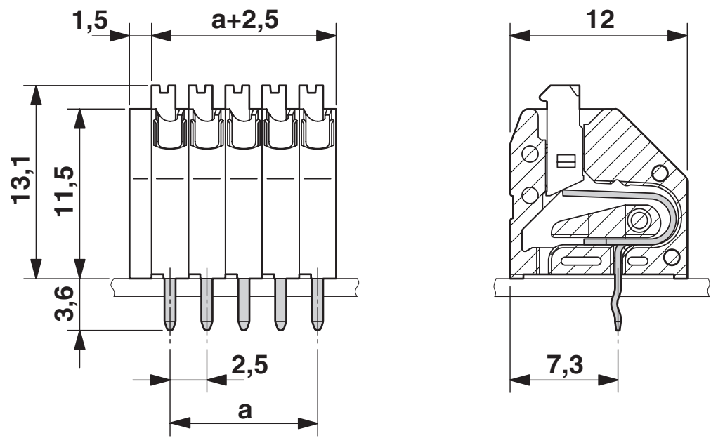
尺寸图
