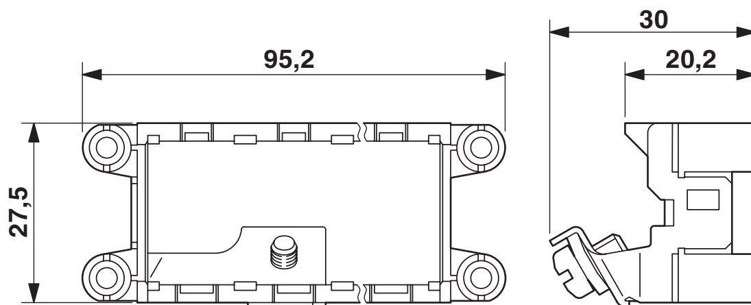
尺寸图
