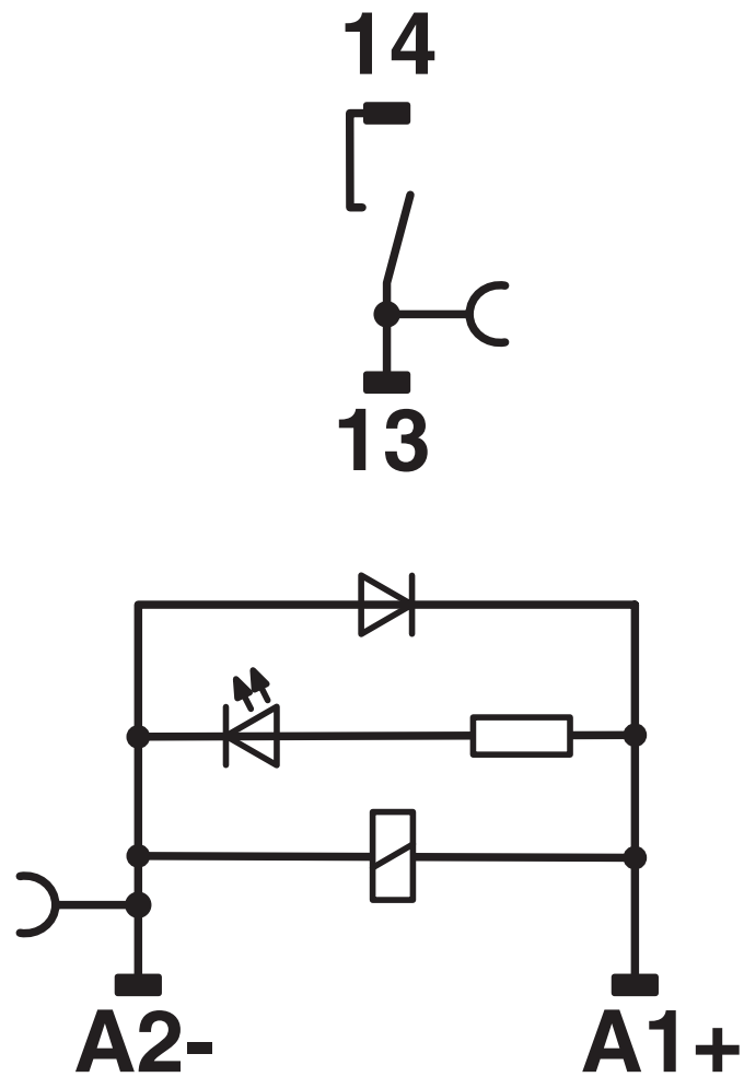
电路图
