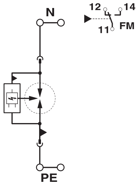
电路图
